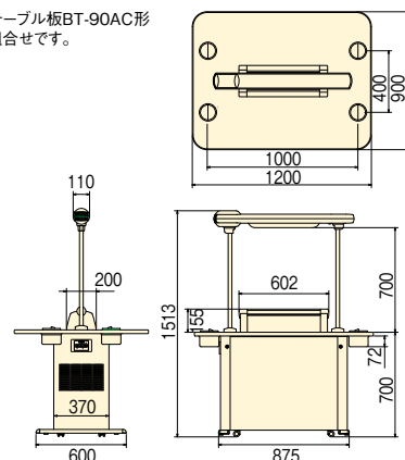
カウンタータイプ BS-C13C 組合せ寸法図 (mm)
